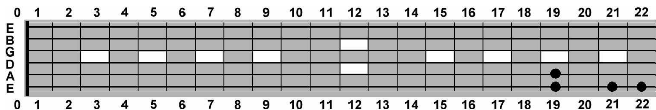
RE Maggiore 18 Posizione
